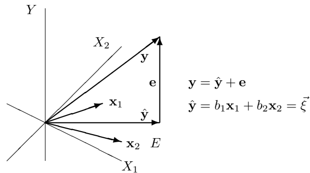
Abbildung 1: \hat{y} als Projektion von y auf C(X)
